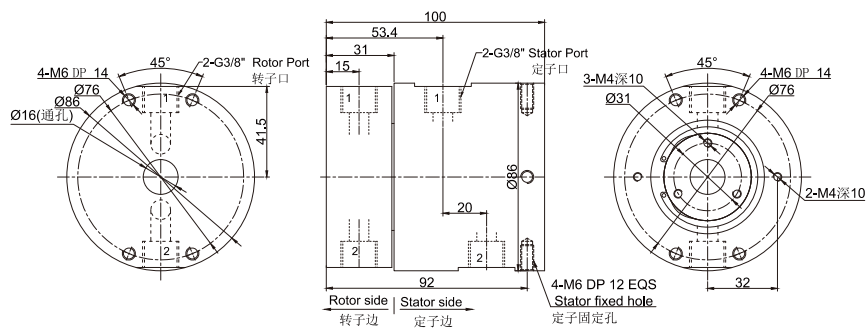
2进2出G3/8"牙
