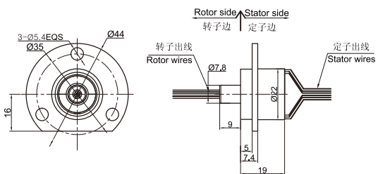
DC190-FL06图片及外形尺寸图
