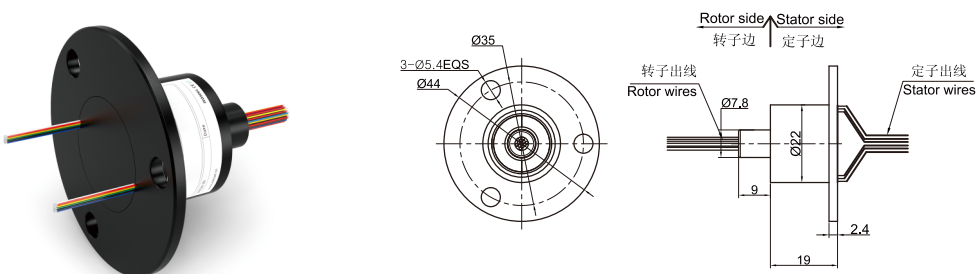
DC190-FL02图片及外形尺寸图
