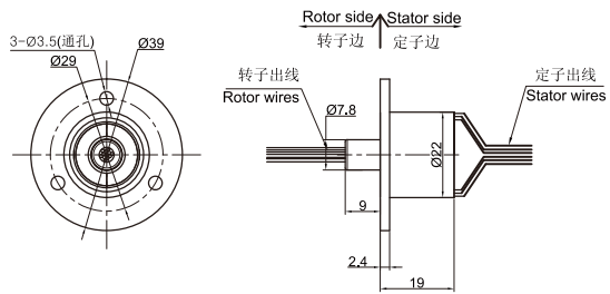
DC190-FL03图片及外形尺寸图
