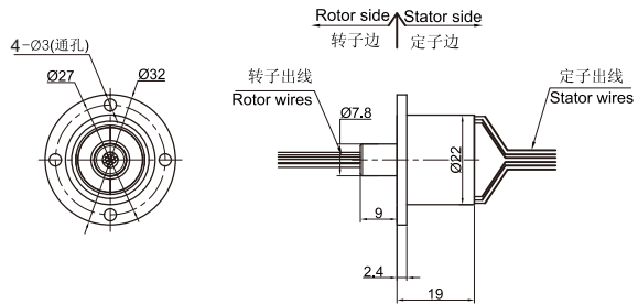
DC190-FL04图片及外形尺寸图
