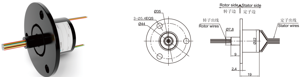
DC190-FL01图片及外形尺寸图
