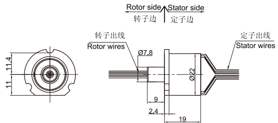
DC190-FL05图片及外形尺寸图
