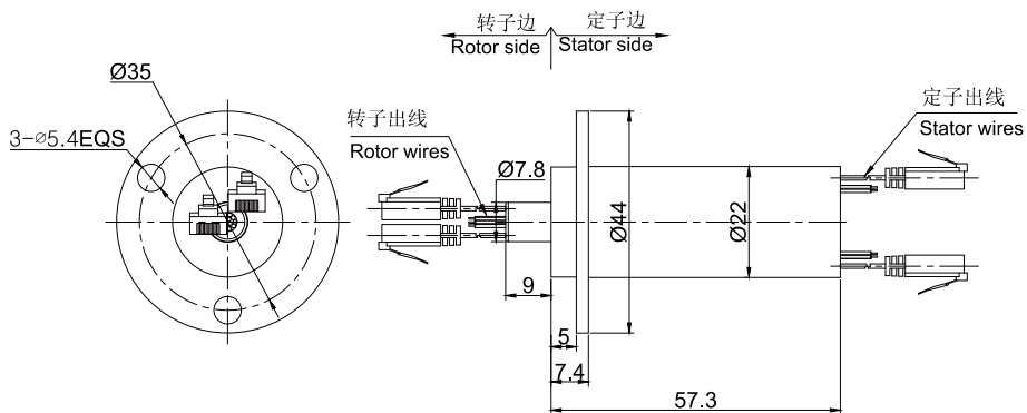
DE1222-S20 外形图尺寸图
