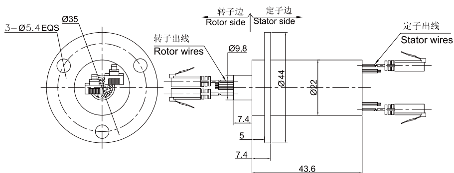
DE1222-S08 外形图尺寸图
