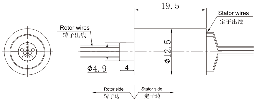
DMC195-FL00外形尺寸图
