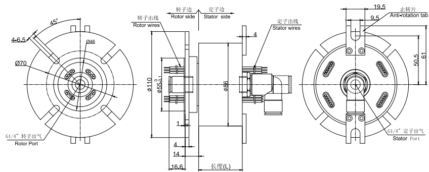
1进1出, G3/8接头 DAPH100-04 尺寸图
