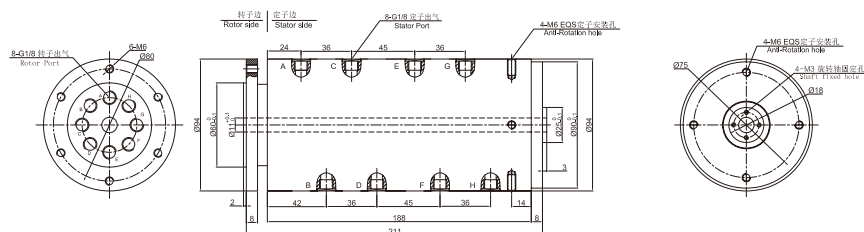
DAPH800-02纯气 尺寸图 ▼
