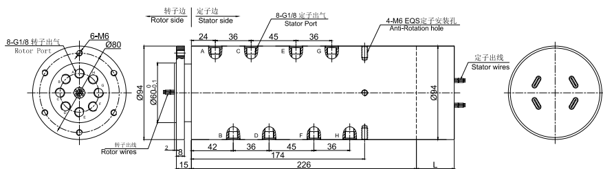
DAFH800-02气电一体 尺寸图 ▼
