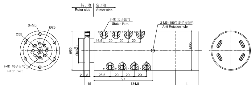
DAFH800-01气电一体 尺寸图 ▼
