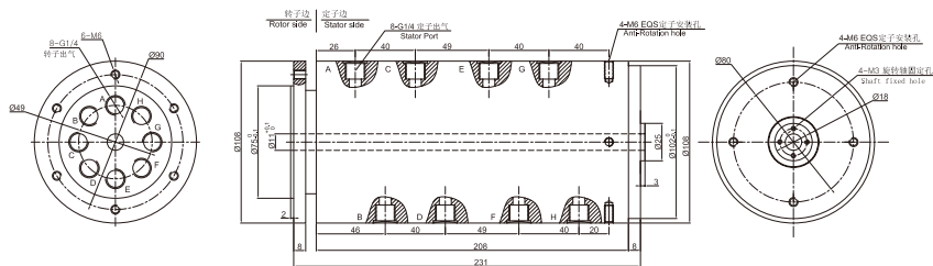
DAFH800-03纯气 尺寸图 ▼
