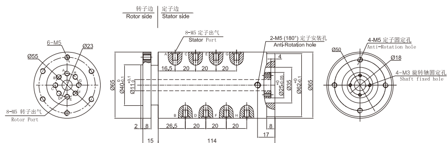
DAPH800-01纯气 尺寸图 ▼
